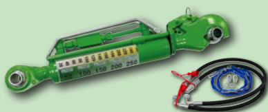
Hydraulischer Oberlenker SAUGUT Kat.2 mit Fanghaken, Kugelaug und Oberlenkerbügel, Hub 250mm
