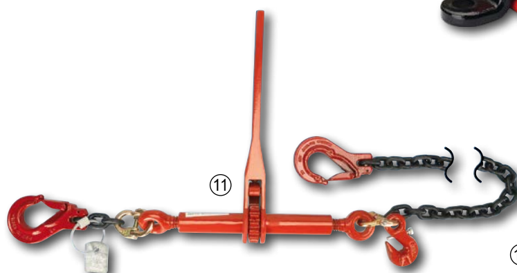
11 Zurrkette mit Ratschenspanner Standardlänge 3 m (+Verstellbereich), mit 2 Sicherheitslasthaken und einem Parallelhaken zum Verkürzen der Kette.
