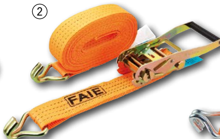
2 Zurrgurt FAIE 50 mm Mit Ratsche mit 2 Rundhaken, Länge 12 m, 50 mm Breite, zul. Zugkraft 2000 daN, in Umreifung 4000 daN. Menge Best. Nr. EUR 1 Garnitur H 32354 24,95 2 Garnituren H 35118 42,90
