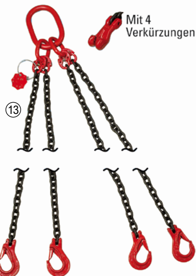
13 Anschlagkette 4-strängig 8 mm, 3 Meter Nutzlänge mit 4 Verkürzungen, mit Ring und Lasthaken, mit Prüfplakette, Tragfähigkeit: bei 45° - 4250 kg, bei 60° - 3000 kg. Best. Nr. H 59366 EUR 339,00
